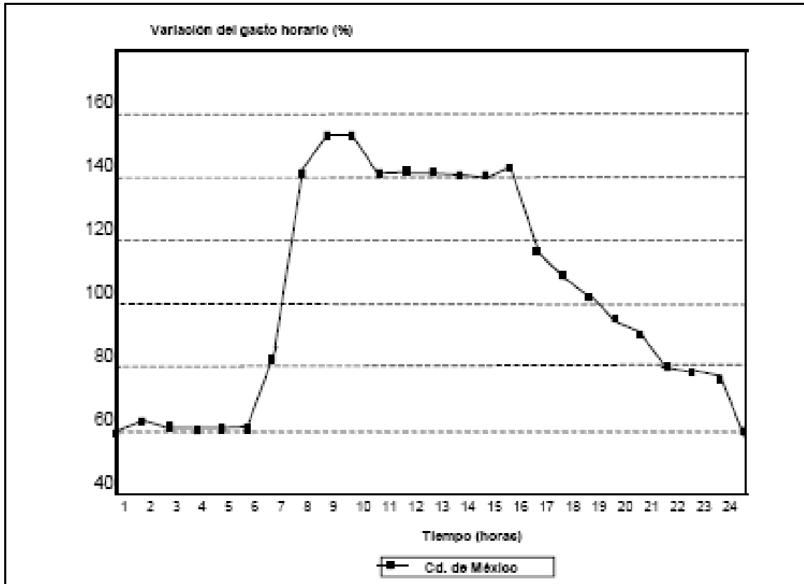
Figura 2.5. Variación del gasto horario en la Ciudad de México (BANOBRAS)
