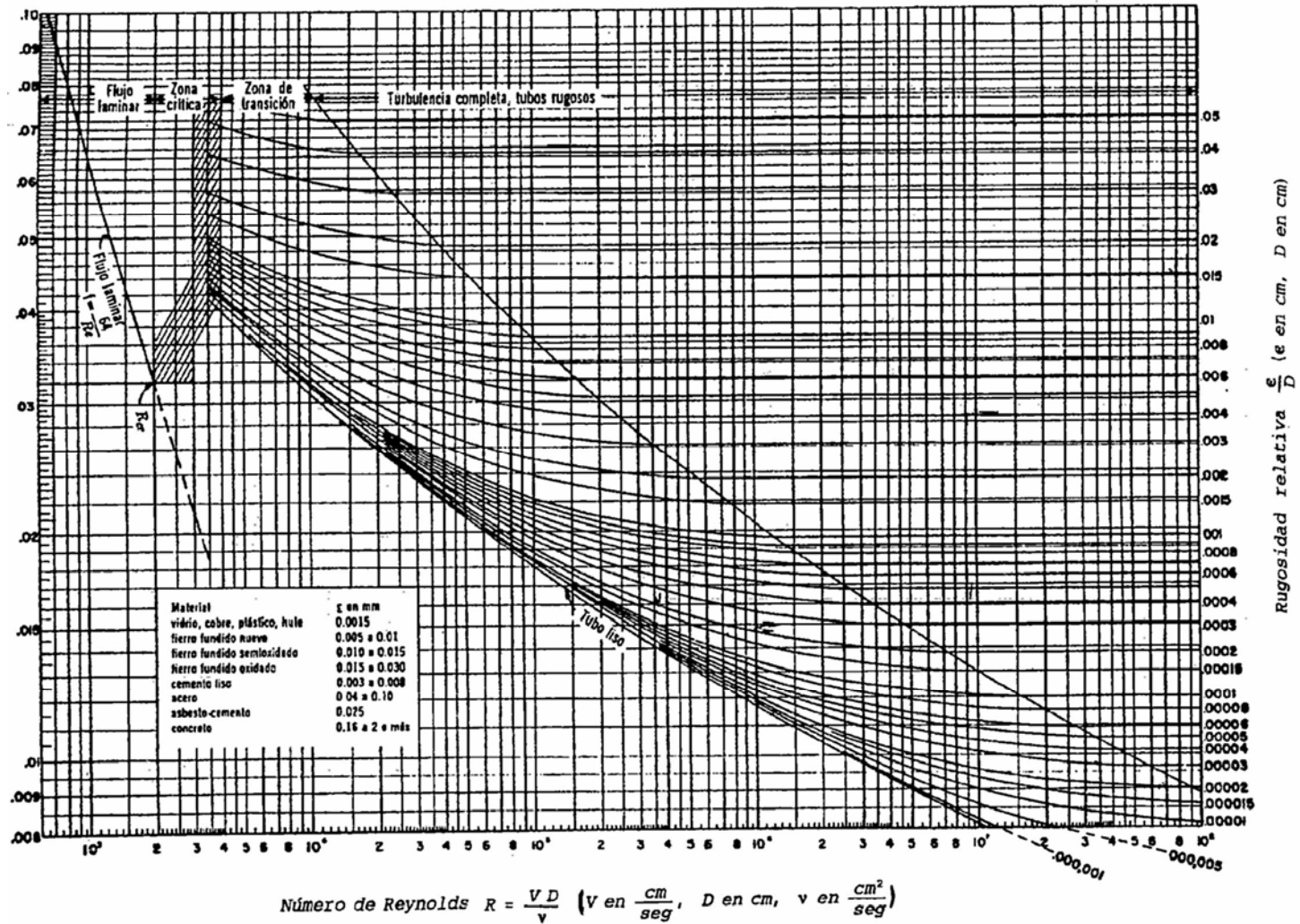
Figura 2.1. Coeficiente de fricción para cualquier tipo y tamaño de tubo. (Diagrama universal de Moody).
