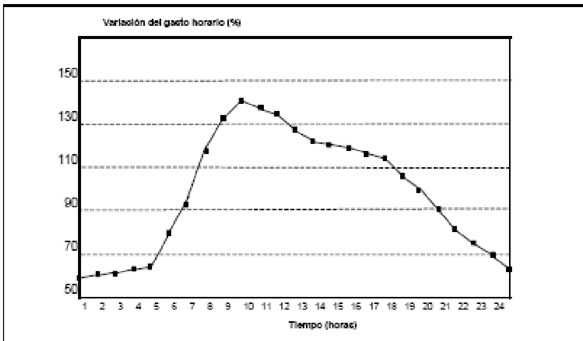
Figura 2.4. Variación del gasto horario (ref. 3)
