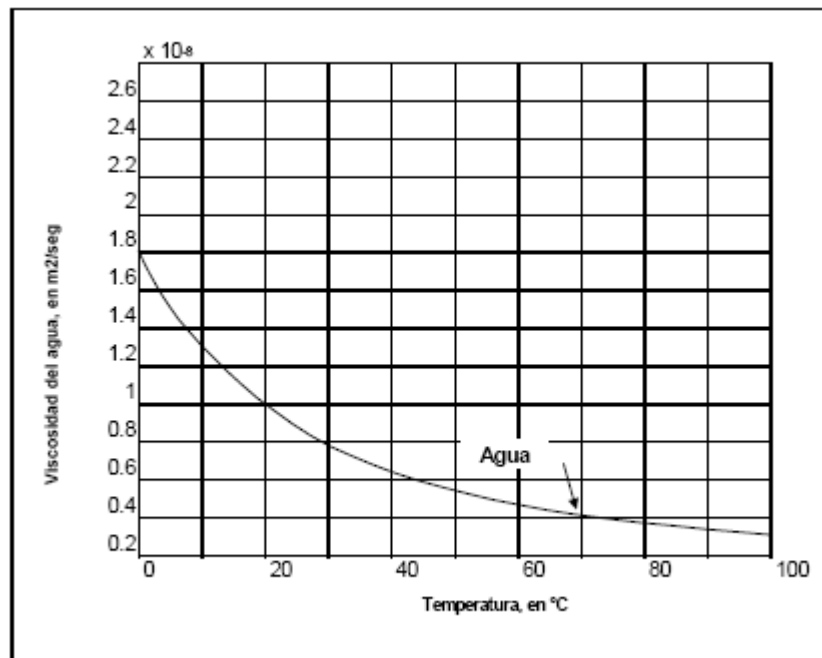
Figura 2.1. Variación de la viscosidad cinemática del agua(ν) con la temperatura (ref. 10)
