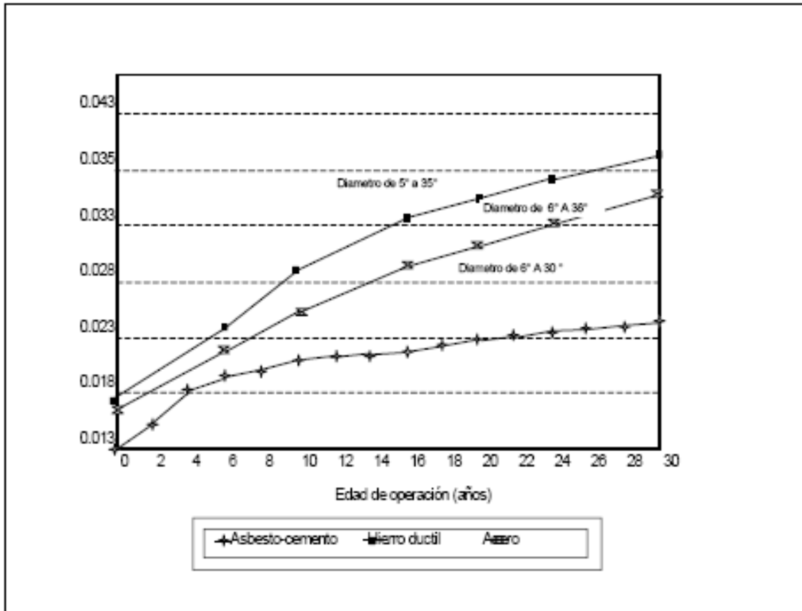
Figura 2.2. Variación del coeficiente de fricción "f" para aplicarse en la fórmula de Darcy, con la edad de la tubería para diferentes materiales.
