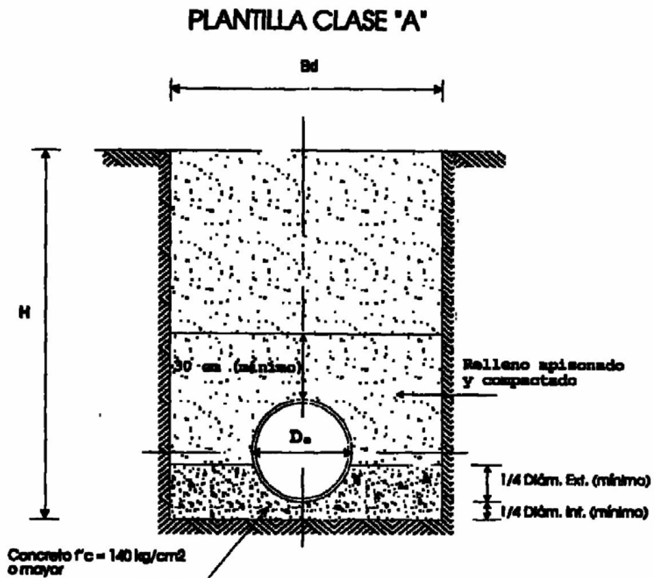
Figura 3.2. Plantilla Clase "A"
