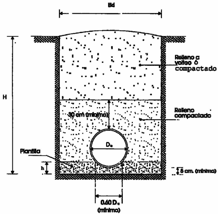
Figura 2.6 Relleno de zanja
