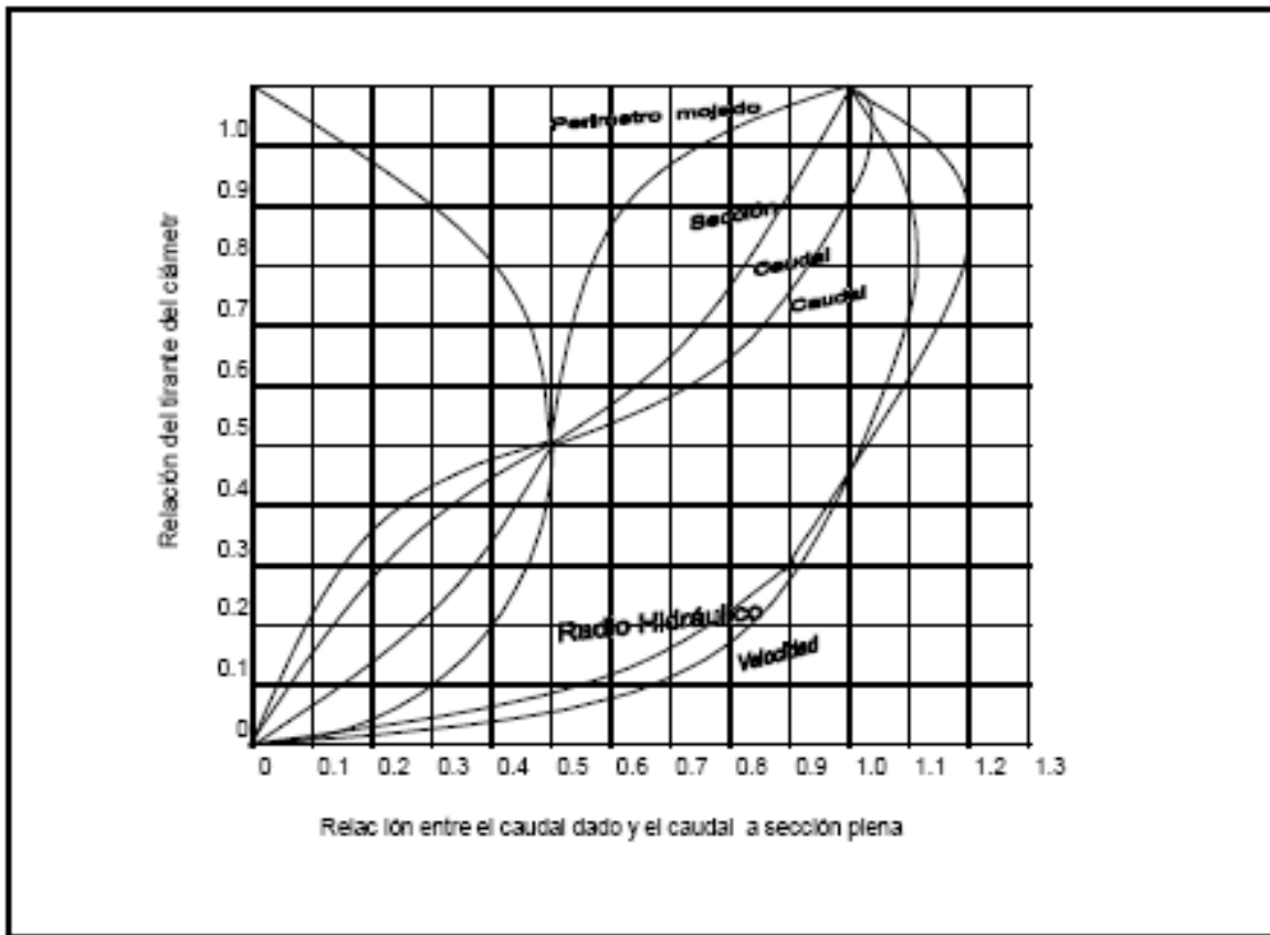
Figura 3.1. Elementos hidráulicos de la sección circular.
