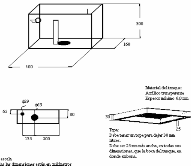
FIGURA 2 DIMENSIONES BASICAS DEL TANQUE DE PRUEBA
