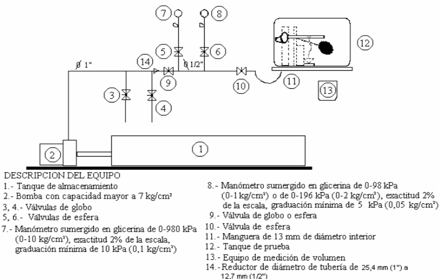
FIGURA 1. EQUIPO DE PRUEBA
