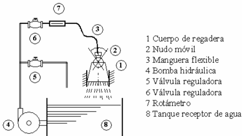
Figura 5. Instalación de prueba
