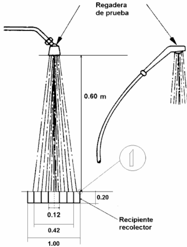
Figura 3. Eficiencia de la regadera
