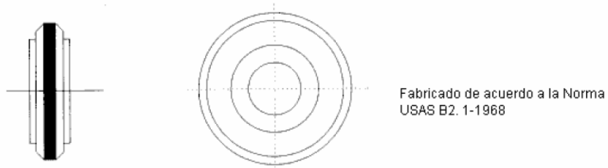
Figura 4. Calibrador hembra
