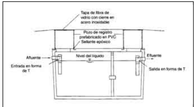
Figura 1 Fosa séptica moderna.
