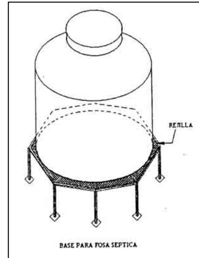
Figura 6 Base para fosa séptica.
