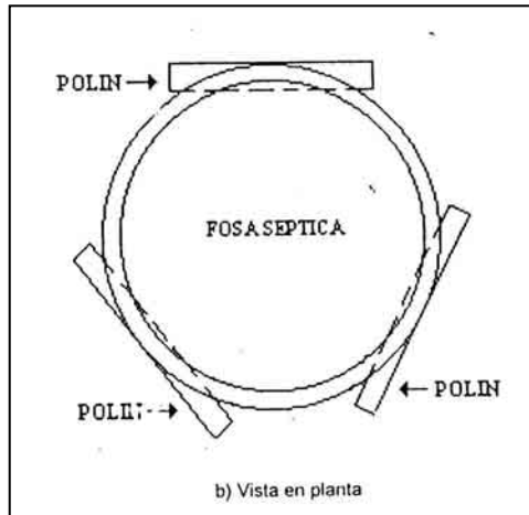
Figura 5 Colocación de fosa séptica sobre polines de madera.
